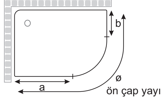
SOL ASİMETRİK OVAL DUŞ TEKNESİ VE KÜVET ÖLÇÜLENDİRME
