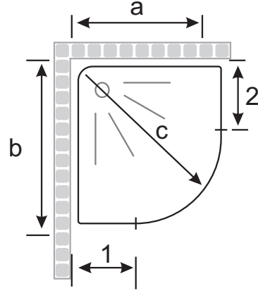
OVAL DUŞ TEKNESİ VE KÜVET YANLARI DÜZ ÖLÇÜLENDİRME
