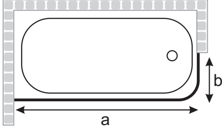
KÜVET ÜSTÜ ÖN CEPHE KENAR ÖLÇÜLENDİRME
