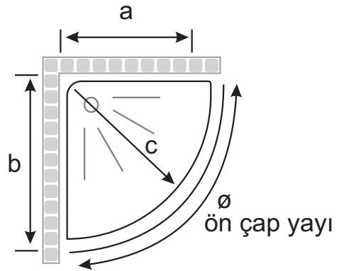
OVAL DUŞ TEKNESİ VE KÜVET ÖLÇÜLENDİRME
