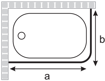
OTURMALI KÜVET 105'LİK İKİ KENAR ÖLÇÜLENDİRME
