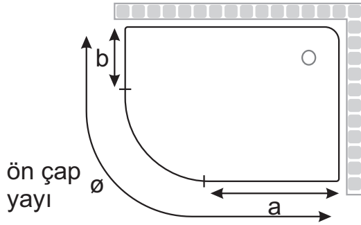
SAĞ ASİMETRİK OVAL DUŞ TEKNESİ VE KÜVET ÖLÇÜLENDİRME
